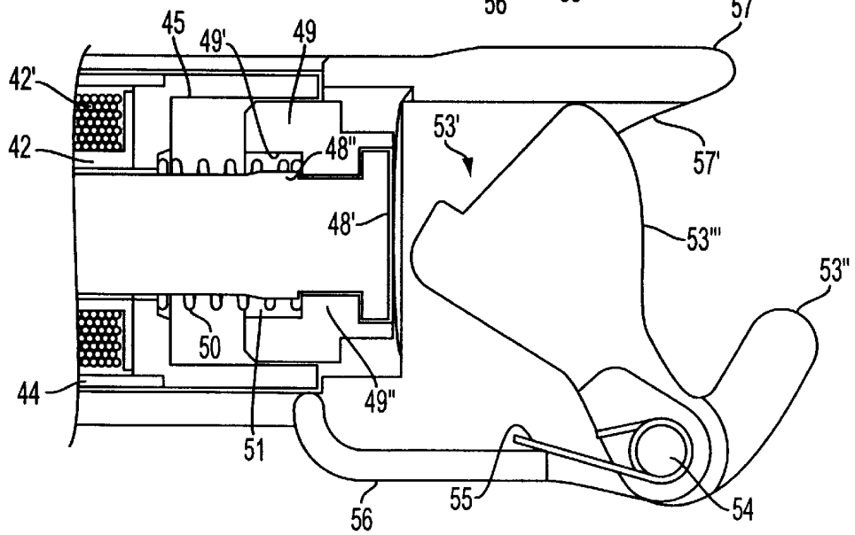
FIG. 13E
