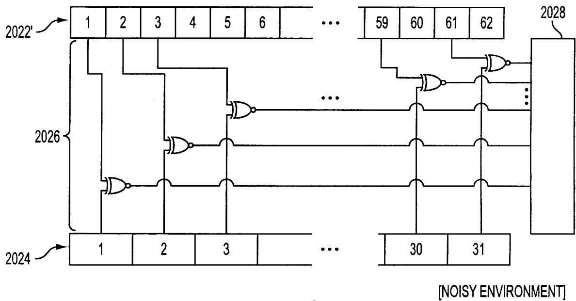
FIG. 15B
