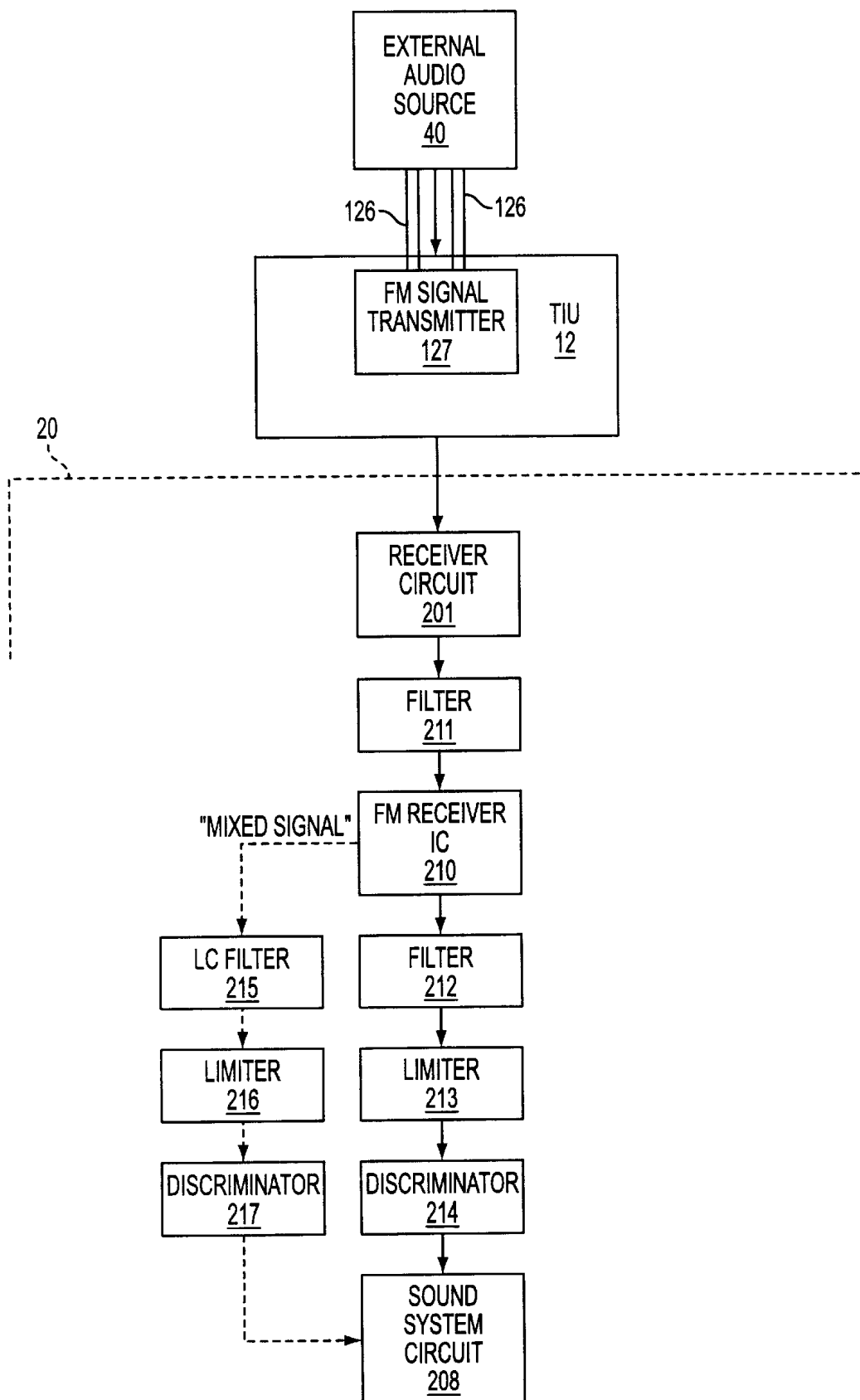
FIG. 4A
