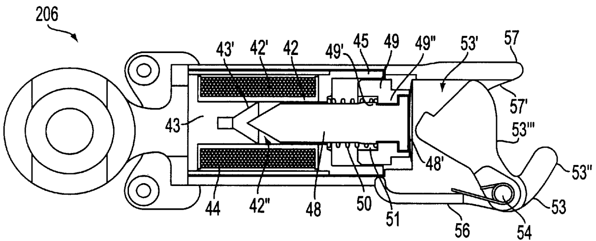
FIG. 13C
