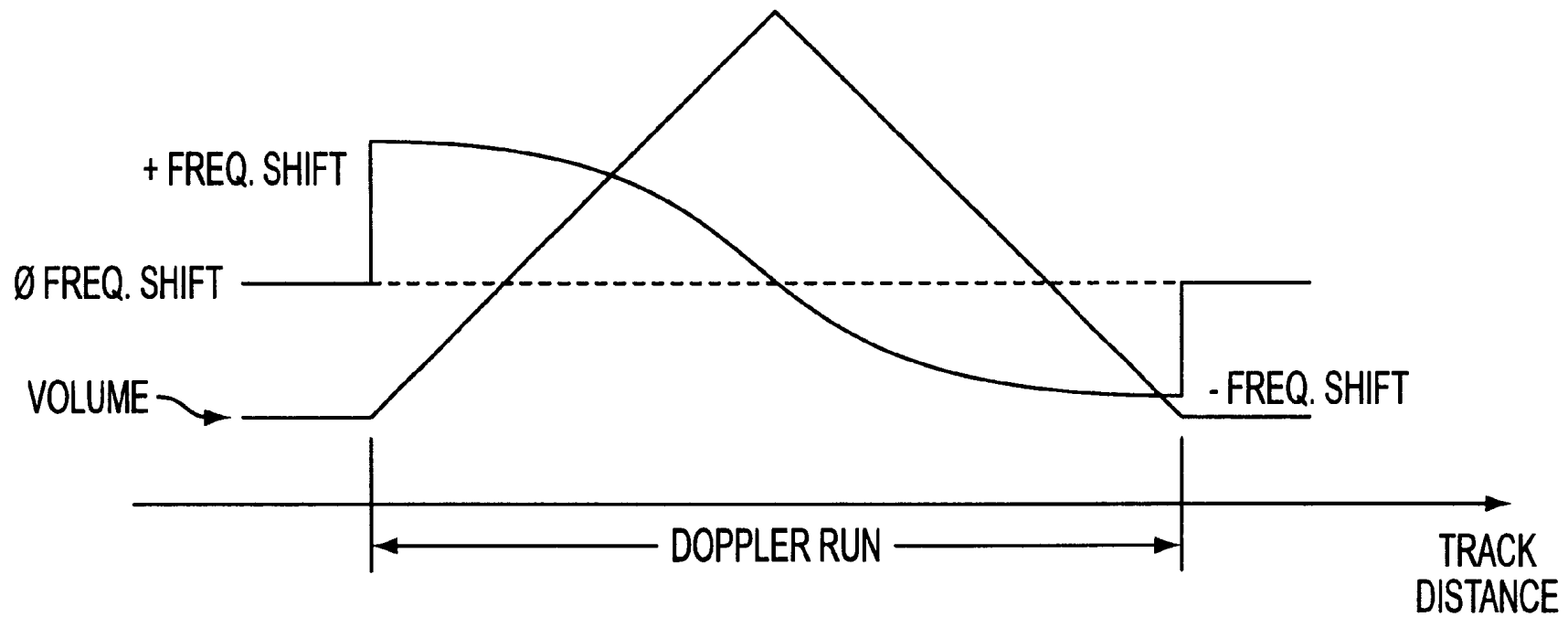
FIG. 16D
