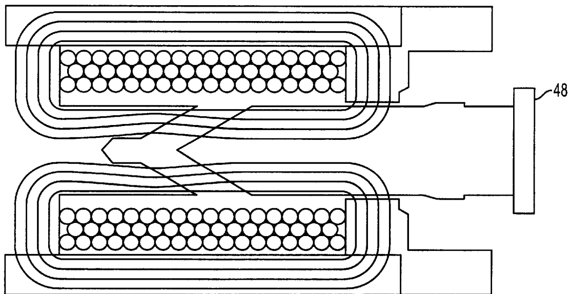
FIG. 13G
