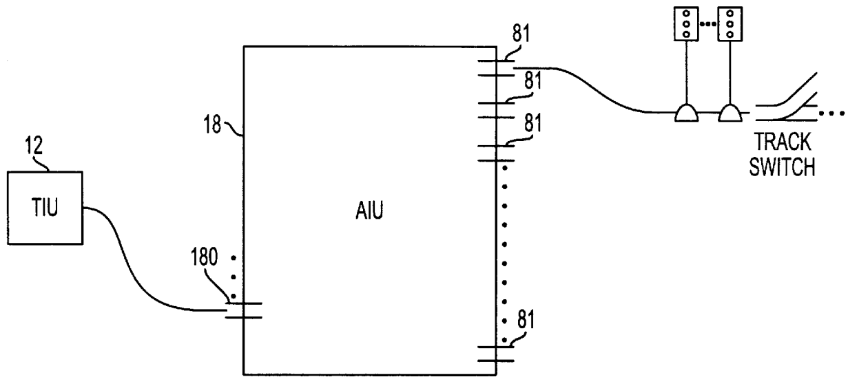
FIG. 17A
