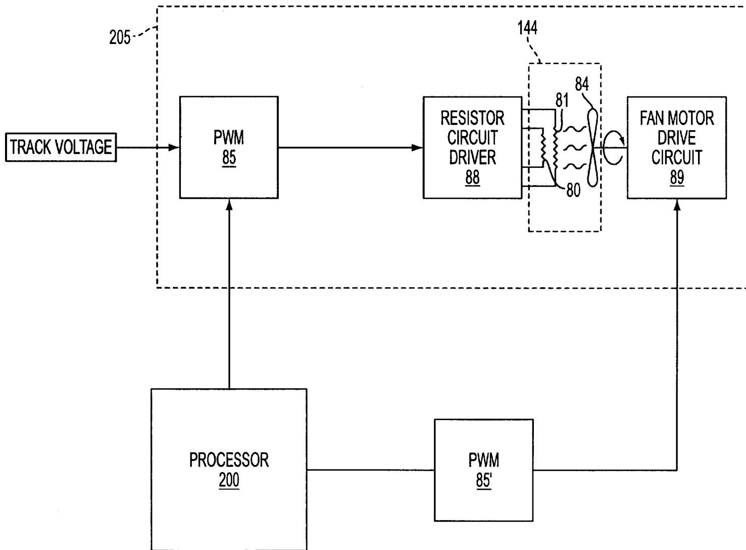
FIG. 14C
